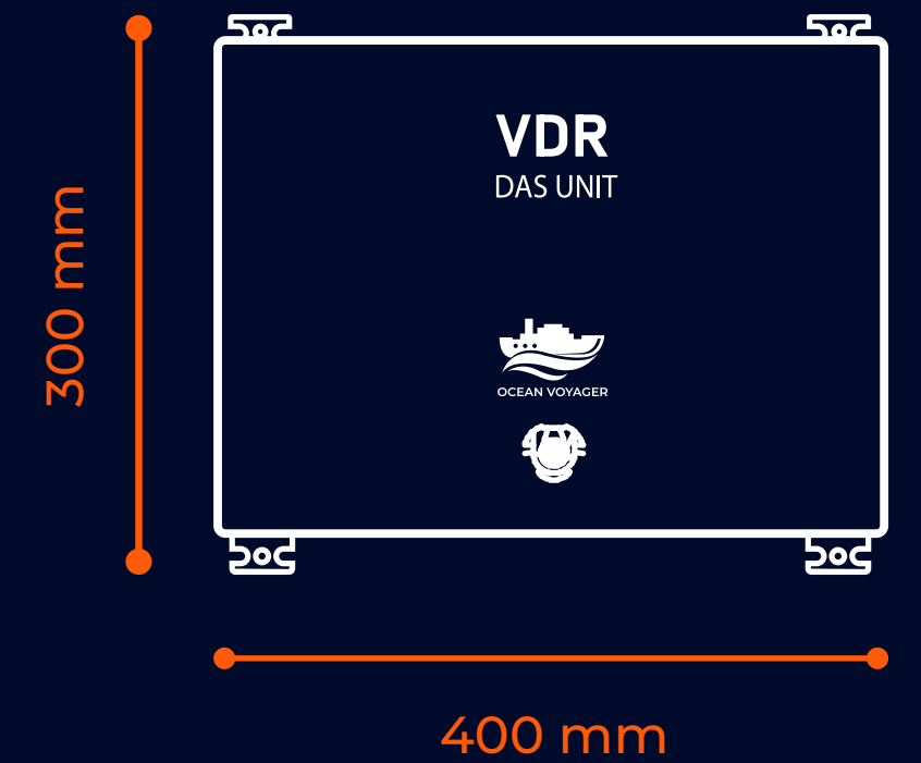
Digital-Analog-Serial Unit
